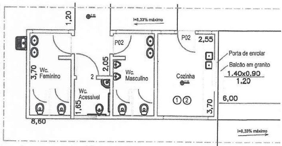
PLANTA BAIXA- Lanchonete externa Sem escala
