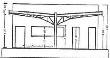
CORTE B:B Escala: 1:100
